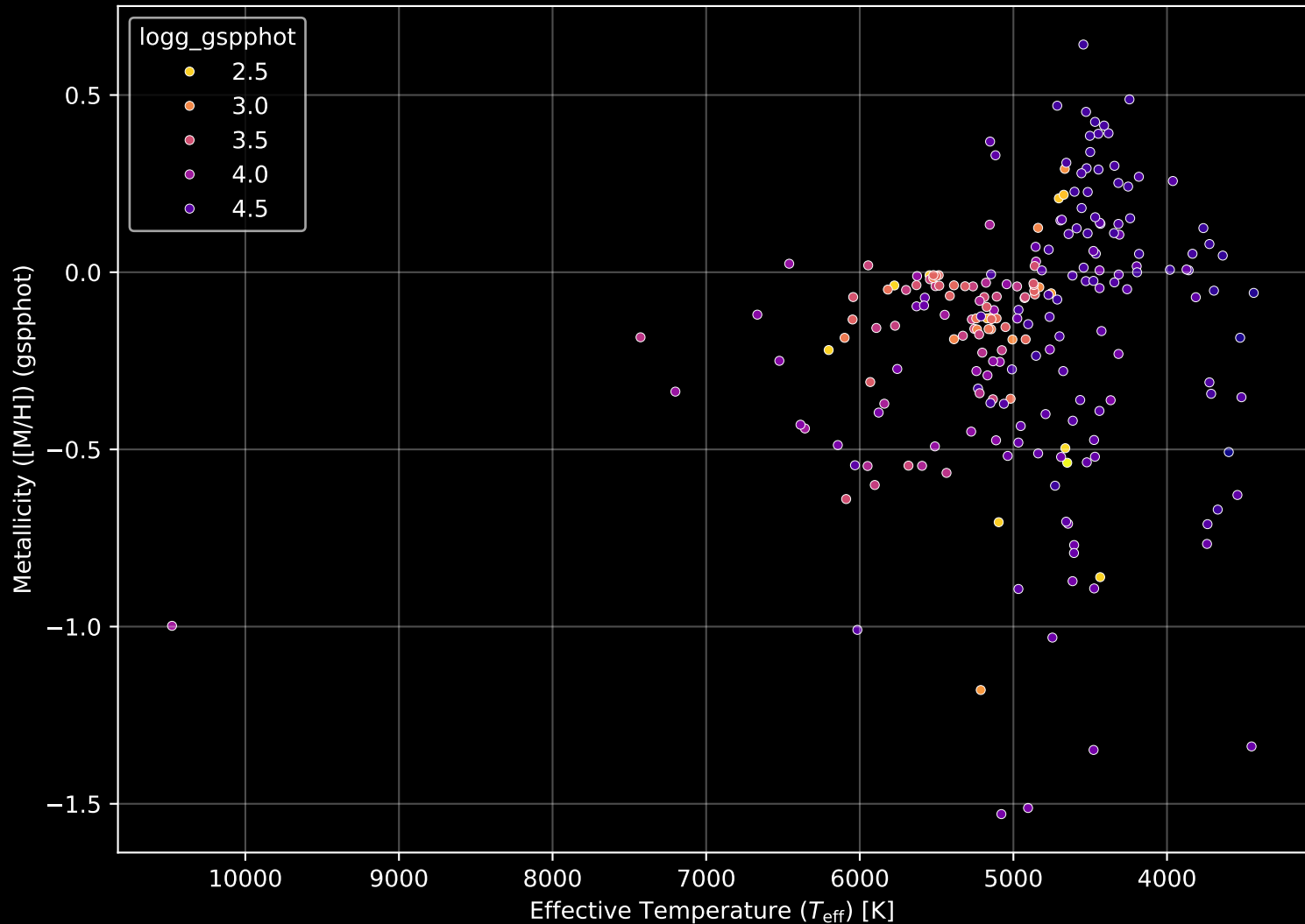
APOGEE DR17 Field: [301-33-C] Stellar Population Parameters (n= 221)
